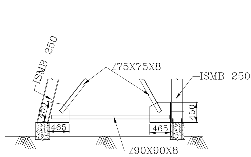
DETAIL-D (SCALE- 1:50)
