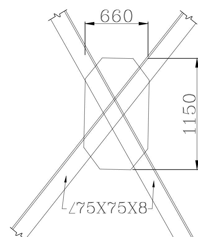
DETAIL: X' (SCALE- 1:25)
