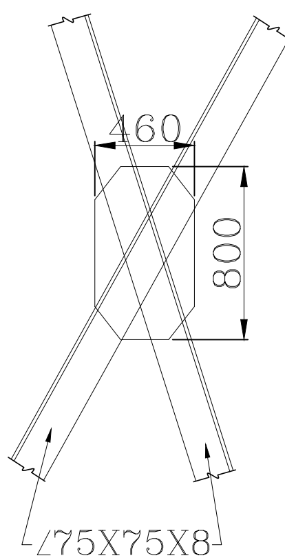
DETAIL: Y' (SCALE- 1:25)
