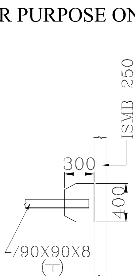
DETAIL: Z' (SCALE- 1:25)
